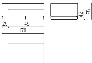
Elemento angolare S.G. o D.G. schienale fisso/ Corner unit left or right fixed backrest
