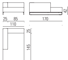
Dormeuse terminale S.G. o D.G. schienale fisso/ End long chair left or right fixed backrest
