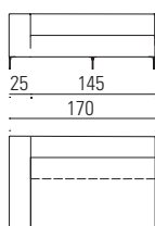
Terminale S.G. o D.G./ End unit left or right/ 170
